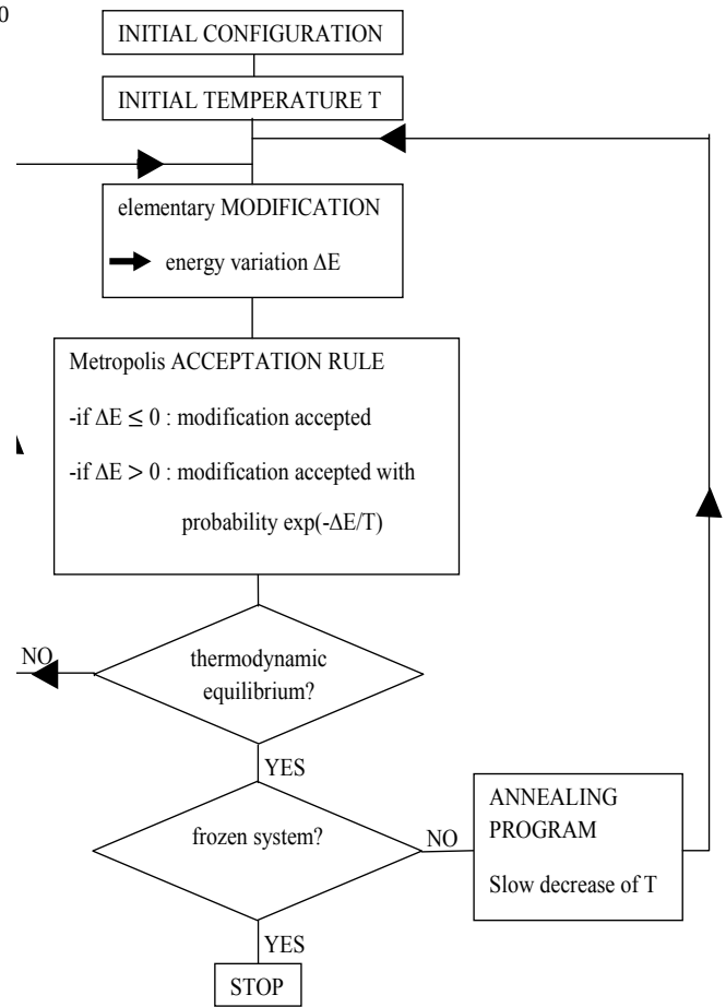
Fig. 2. Flowchart of SA [10].
